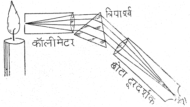
चित्र १६—रश्मि-विश्लेषक यंत्र की बनावट। [ सौर-परिवार से ]
